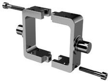
Charnela para cilindros de perfil mod. F-63
