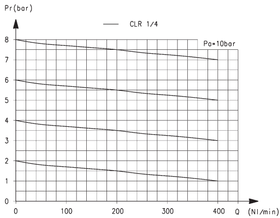
G1/4 接口铰接式微型减压器流量特性曲线
