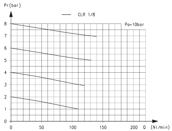
G1/8 接口铰接式微型减压器流量特性曲线
