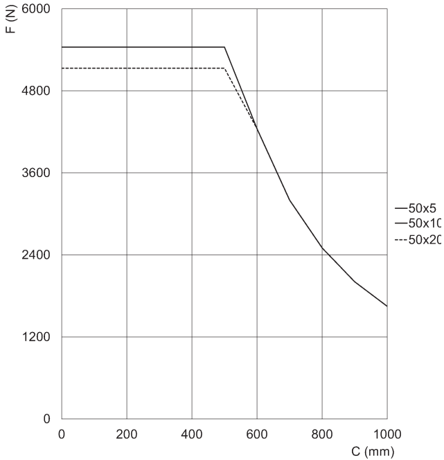
Baugröße 50 mm
