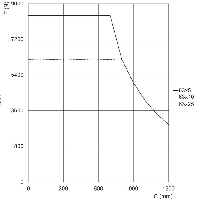
Baugröße 63 mm
