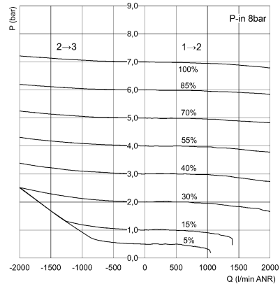
Curva caratteristica della versione PRE204-xG..
