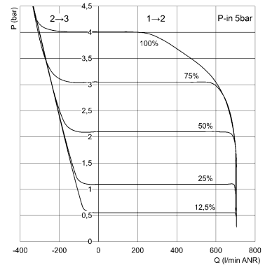
Curva caratteristica della versione PRE104-xE..
