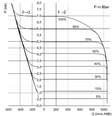
Curva caratteristica della versione PRE104-xG..
