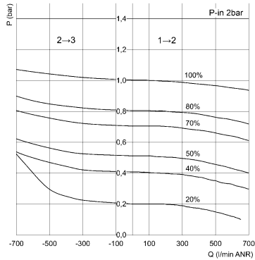
Curva caratteristica della portata da 0,2 a 1 bar
