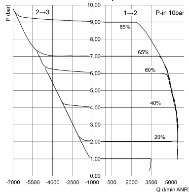
Curva caratteristica della portata da 1 a 9 bar
