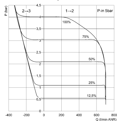
Curva caratteristica della portata da 0,5 a 4 bar
