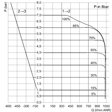
Curva caratteristica della portata da 0,5 a 7 bar
