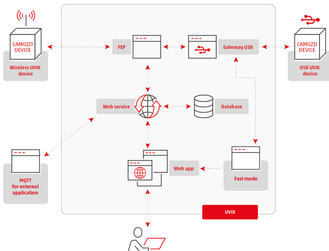
Figura 3.1: Struttura dell'UVIX
