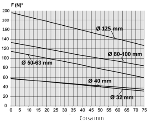
Serie 63 - molla anteriore
