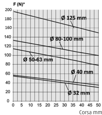
Serie 63 - molla posteriore
