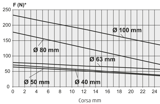
Serie 63 - molla anteriore
