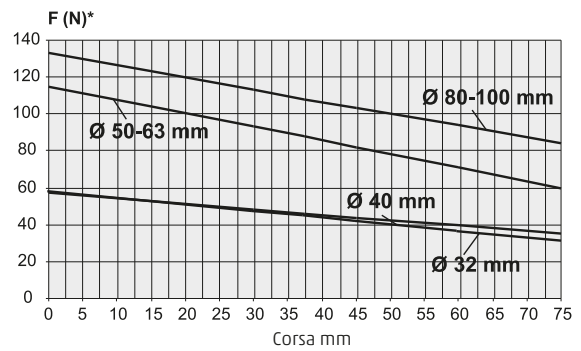
Serie 63 - molla posteriore
